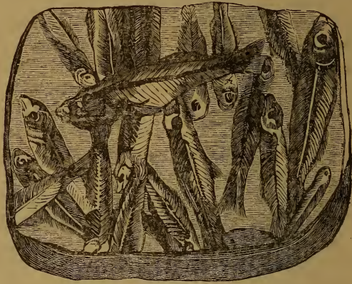
Fig. 16.—Fossil Fish from Aix
